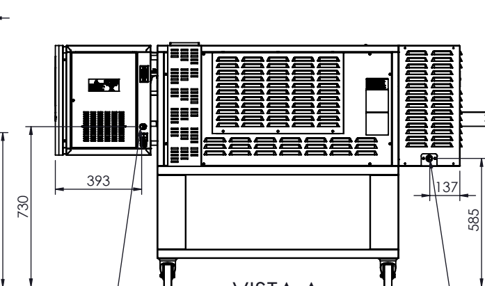
ingresso alimentazione gas / gas supply entry -
