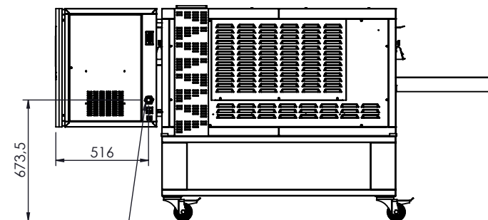
VISTA A
