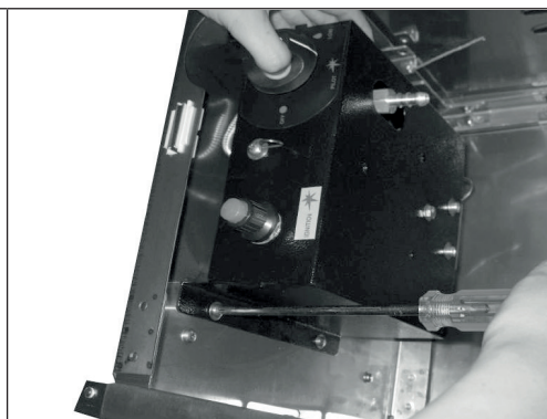
ETAPA 2: Carcasa rezervorului se menține în poziție culcată. Se montează ansamblul arzătorului (J) pe carcasa rezervorului folosind 4 buc de șuruburi și piulițe standard (BB).
