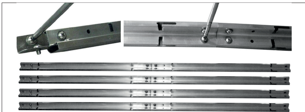
ETAPA 3: Se deșurubează cele 2 buc de șuruburi și piulițe standard (BB) de pe bara de sprijin - inferioară (F). Se introduce bara de sprijin superioară (E) în bara de sprijin - inferioară (F) și se fixează cu cele 2 buc de șuruburi și piulițe standard (BB). Acest pas se repetă la conectarea celor 3 seturi de bare de sprijin.
